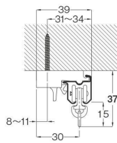
天井付シングルブラケット付 (ブラケット幅=32mm)
