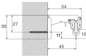
LTダブルブラケット付 (ブラケット幅=35mm)
