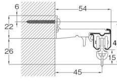
エキストラシングルブラケット付 (ブラケット幅=18mm)
