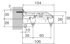
カバートップⅡセット側面図
