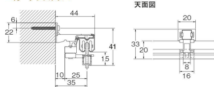
カバートップⅡセット平面図
