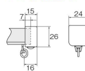
カバートップⅡセット側面図
