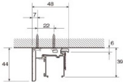
天井付け
