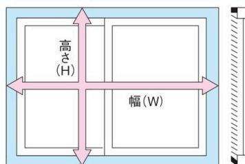
連窓時の必要隙間寸法
