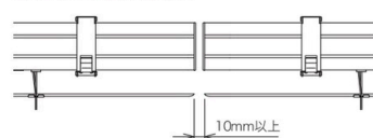
連窓時の必要隙間寸法
