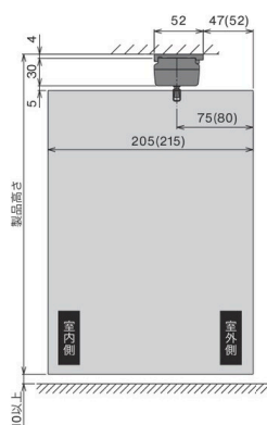
天井付け（ブラケット付け）
