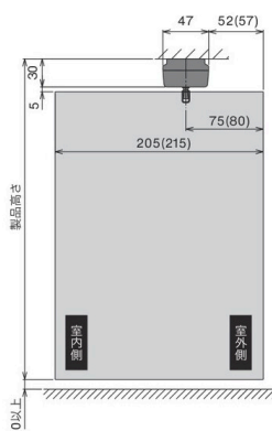
天井付け（直付け）
