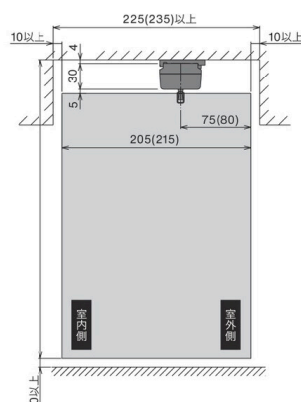
天井付け （カーテンボックス内）
