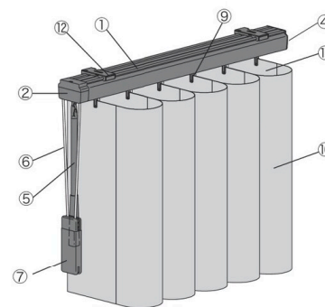
コードウェイト
