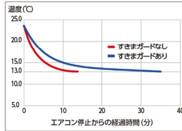
室内の温度推移
