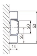
標準取手用
