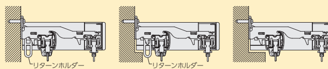
リターンホルダーを付ける
