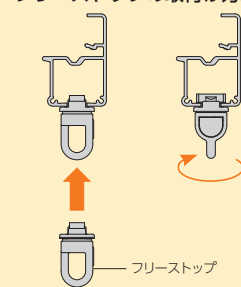
①カーテンエンドの位置にセットする ②フックを90度回転して固定
