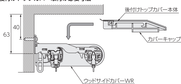
後付けトップカバー取付け必要寸法
