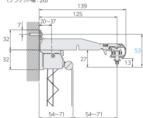
マルチブラケットM+プリーツスクリーン ペルレ(コード操作) (ブラケット幅:26)
