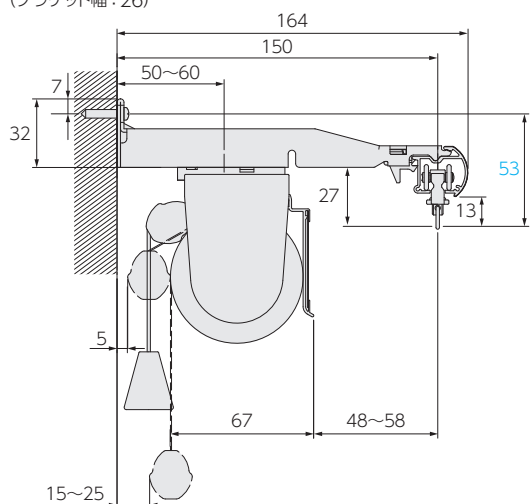
マルチブラケットL+ロールスクリーン ラルクシールド [額縁なし] (ブラケット幅:26)
