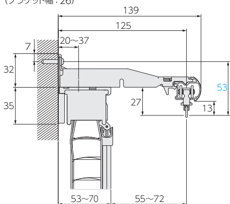
マルチブラケットL+ロールスクリーン ラルクシールド [額縁なし] (ブラケット幅:26)
