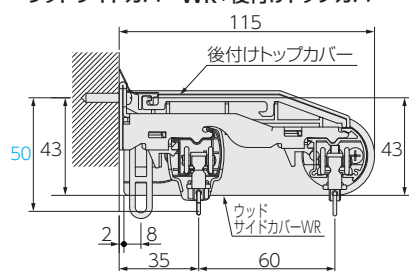
ウッドサイドカバーWR+後付けトップカバー 見下図
