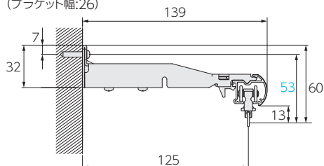
マルチブラケットM (ブラケット幅:26)
