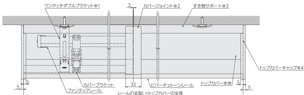
トップカバー 見下図
