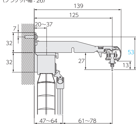
マルチブラケットL+ロールスクリーン ラルクシールド [額縁あり] (ブラケット幅:26)
