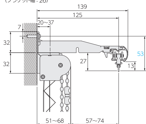
マルチブラケットM+プリーツスクリーン ペルレ(チェーン操作) (ブラケット幅:26)
