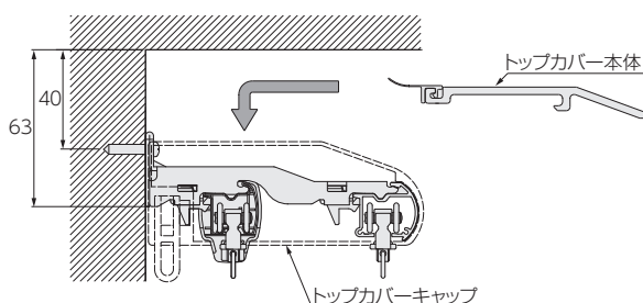
トップカバー取付け必要寸法
