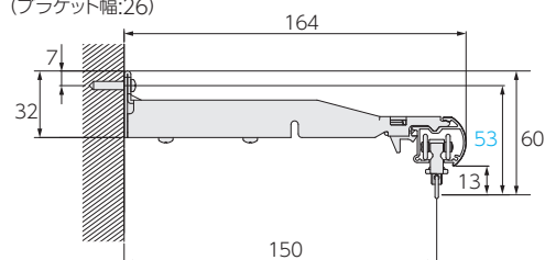
マルチブラケットL (ブラケット幅:26)
