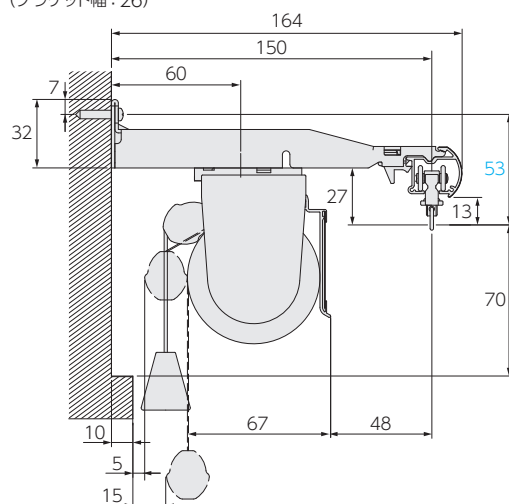
マルチブラケットL+ロールスクリーン ラルクシールド [額縁あり] (ブラケット幅:26)
