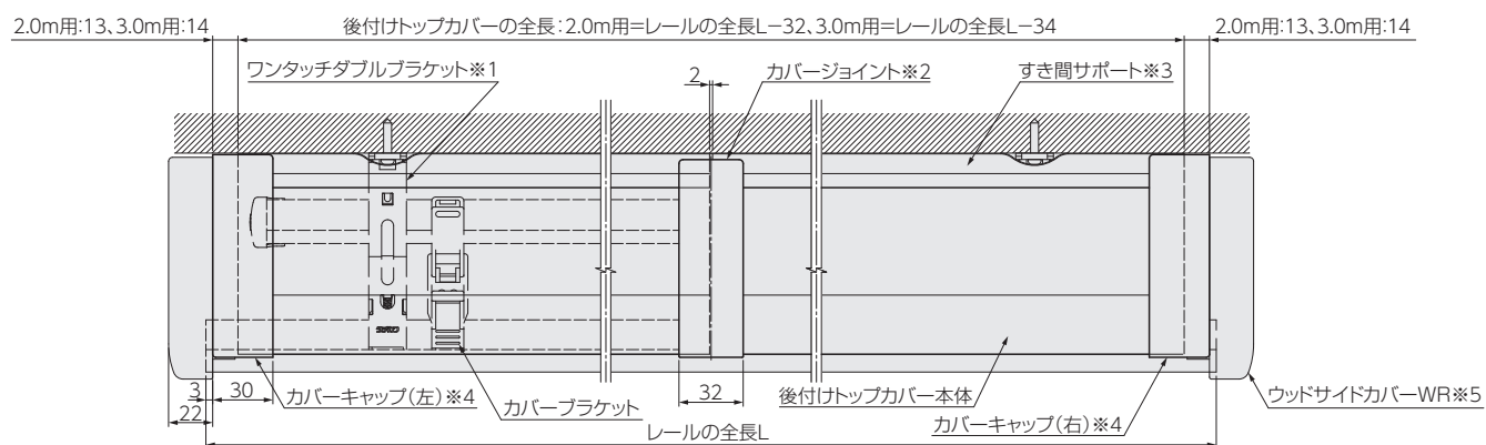
ウッドサイドカバーWR+後付けトップカバー 見下図
