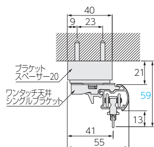
ワンタッチ天井シングルブラケット+ブラケットスペーサー (ブラケット幅：18/ブラケットスペーサー幅：25)
