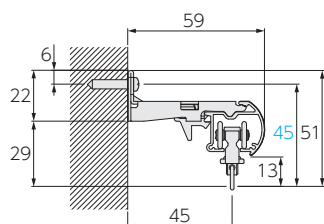
ワンタッチロングシングルブラケット (ブラケット幅：18)
