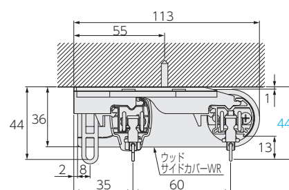
天井ダブルブラケット+ウッドサイドカバーWR
