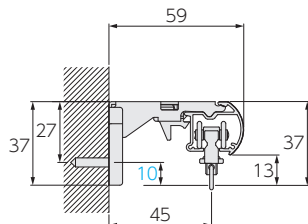
ワンタッチL型シングルブラケット (ブラケット幅：32)
