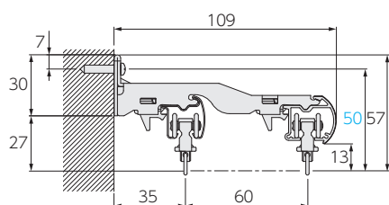
ワンタッチダブルブラケット (ブラケット幅：18)
