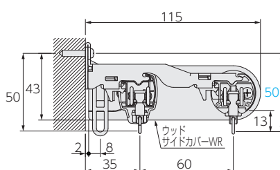
ワンタッチダブルブラケット+ウッドサイドカバーWR
