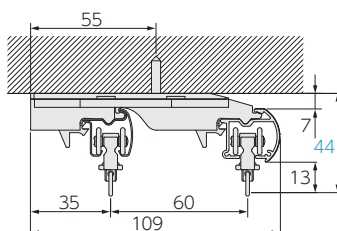
天井ダブルブラケット (ブラケット幅：25)
