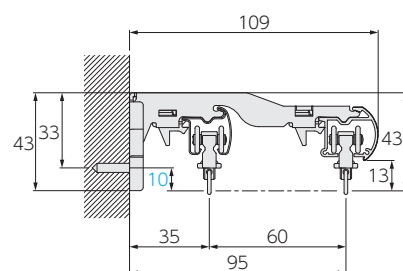
ワンタッチL型ダブルブラケット (ブラケット幅：32)
