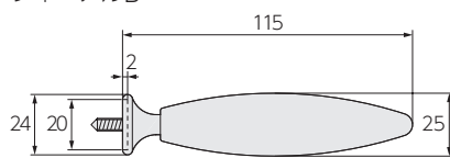
フィニアルB
