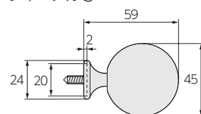
フィニアルC
