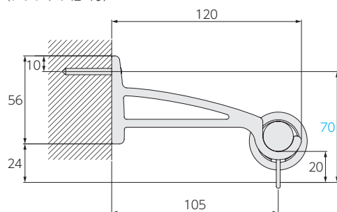
ロングシングルブラケットN (ブラケット幅:19)
