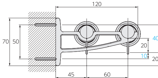
ダブルブラケット (ブラケット幅:19)
