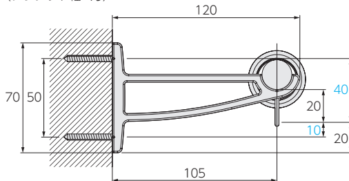
ロングシングルブラケット (ブラケット幅:19)
