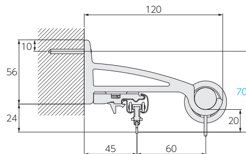
ダブルブラケットN (ブラケット幅:19)
