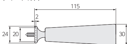
フィニアルA
