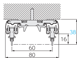
ワンタッチ天井 ダブルブラケット (ブラケット幅:18)
