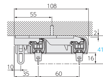
ワンタッチ天井FWブラケット+サイドカバーW
