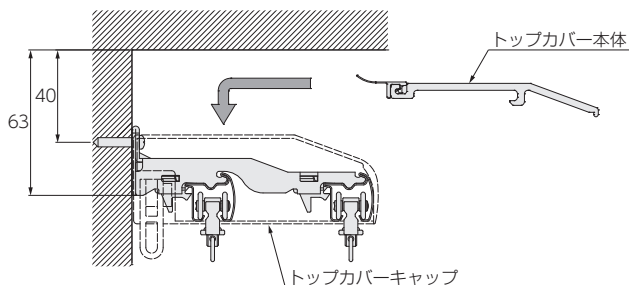
トップカバー取付け必要寸法
