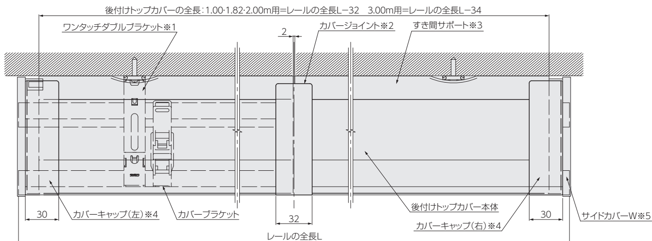
サイドカバーW+後付けトップカバー見下図
