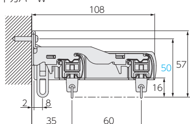
ワンタッチダブルブラケット+ サイドカバーW
