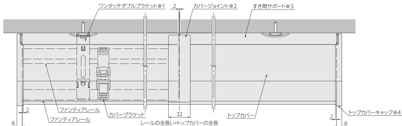
トップカバー見下図
