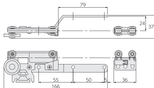
手引き交差ランナー
