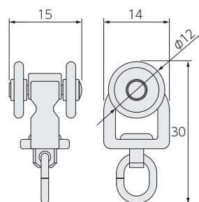
共通ランナー
