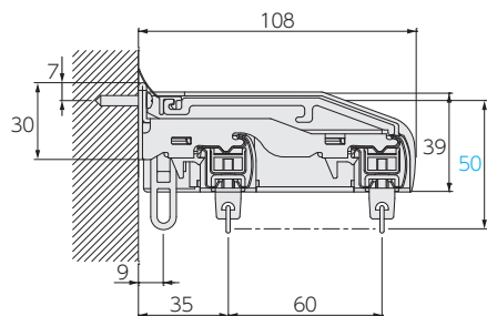
トップカバー見下図
