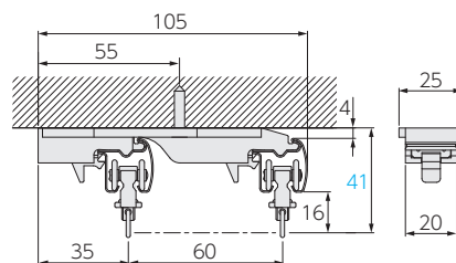
ワンタッチ天井FWブラケット
