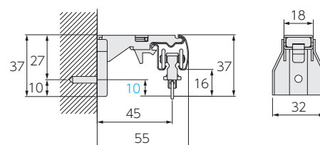
ワンタッチL型シングルブラケット (ブラケット幅:32)
