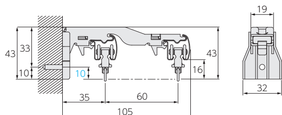
ワンタッチL型ダブルブラケット (ブラケット幅:32)
