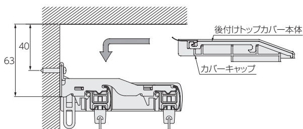
後付けトップカバー取付け必要寸法
