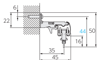
ワンタッチシングルブラケット (ブラケット幅:18)
