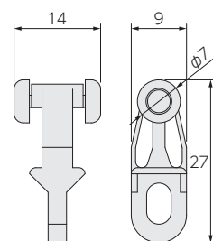
共通後入れランナー
