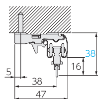
ワンタッチ天井 シングルブラケット (ブラケット幅:18)
