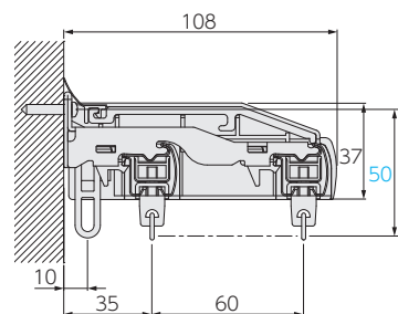
サイドカバーW+後付けトップカバー見下図
