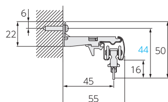
ワンタッチロングシングルブラケット (ブラケット幅:18)
