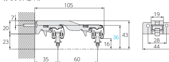
ワンタッチT型ダブルブラケット (ブラケット幅:44)
