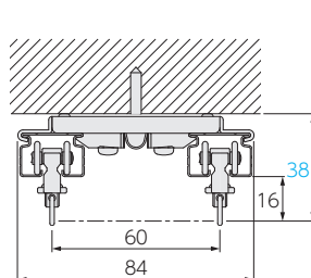
ダブル天井ブラケット (ブラケット幅: 20)
