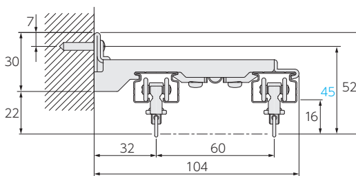
ワンタッチロングダブルブラケット (ブラケット幅: 25)
