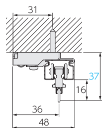
シングル天井ブラケット (ブラケット幅: 20)
