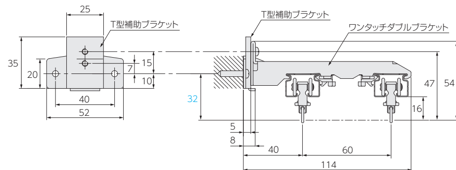
ワンタッチダブルブラケット+T型補助ブラケット
