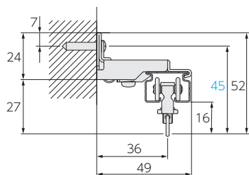
ワンタッチダブルブラケット (ブラケット幅: 21)
