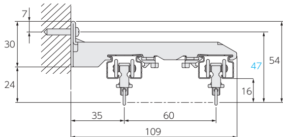
ワンタッチダブルブラケット (ブラケット幅: 21)
