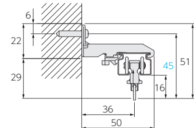
ワンタッチシングルブラケット (ブラケット幅: 20)
