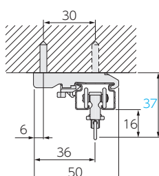
ワンタッチ天井シングルブラケット (ブラケット幅: 20)
