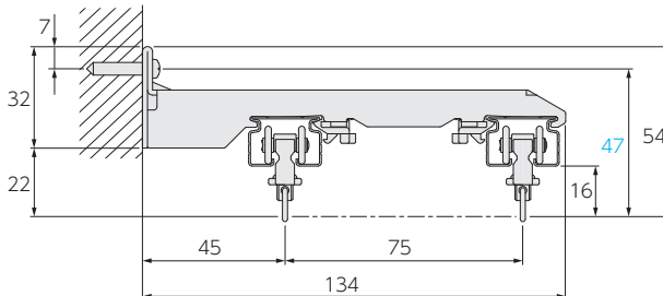
ワンタッチロングダブルブラケット (ブラケット幅: 25)
