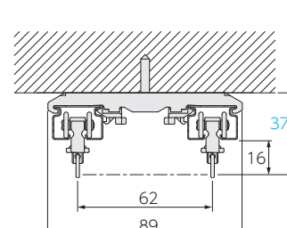
ワンタッチ天井ダブルブラケット (ブラケット幅: 20)
