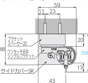
ワンタッチ天井シングルブラケット+ サイドカバーSR (ブラケット幅: 18/ブラケットスペーサー幅: 25)
