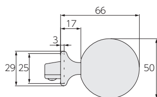
アクセントフィニアルG
