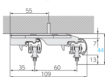
天井ダブルブラケット (ブラケット幅: 25)
