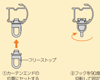
フリーストップをレール端部に付けた場合
