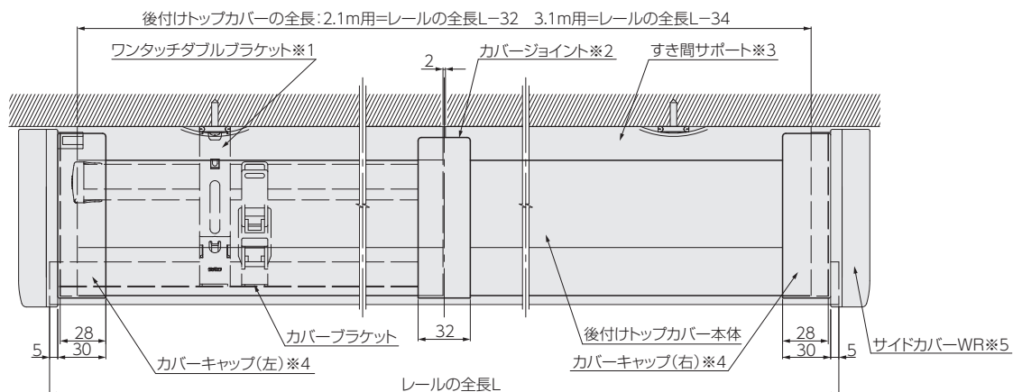
サイドカバーWR+後付けトップカバー 見下図
