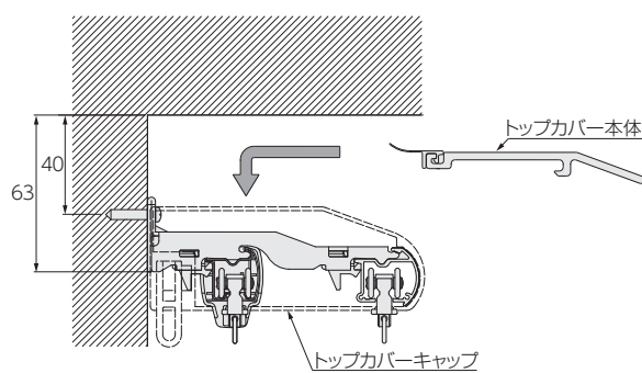
トップカバー取付け必要寸法
