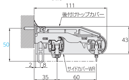
サイドカバーWR+後付けトップカバー
