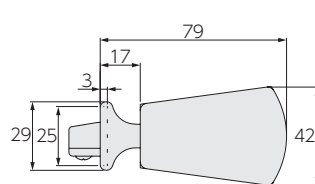
アクセントフィニアルT
