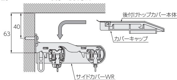
後付けトップカバー取付け必要寸法
