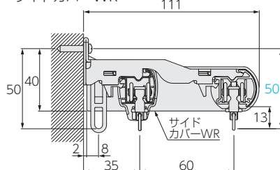
ワンタッチダブルブラケット+ サイドカバーWR
