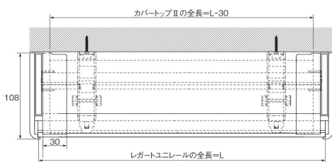
平面图
