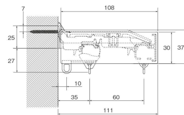
本体側面図
