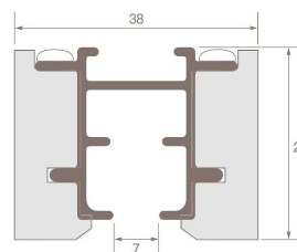
レール断面図 (単位: mm)
