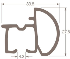
レール断面図（単位：mm）
