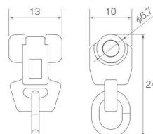
ランナー寸法図 (単位: mm)
