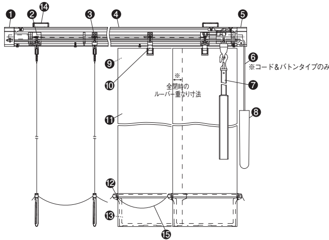
デュアル正面図
