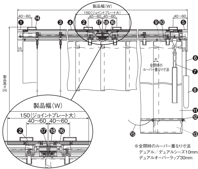
側面図 (mm)
