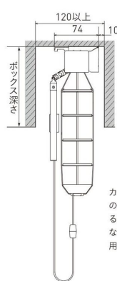
カーテンボックス内 納まり図 (mm)
