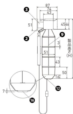
側面図 (mm)
